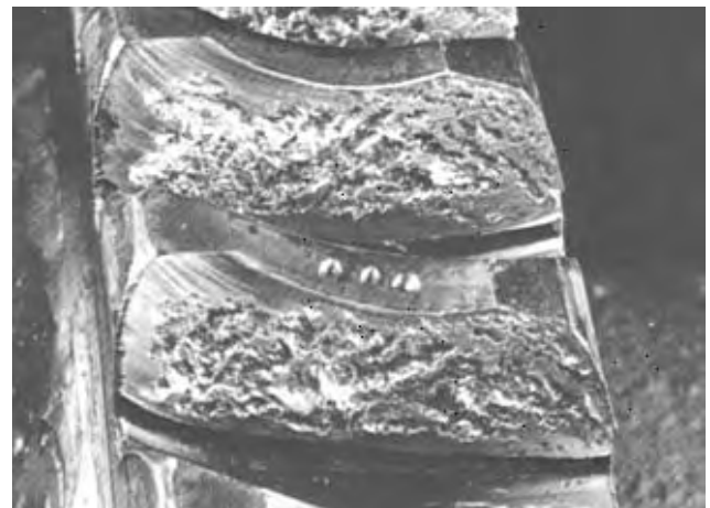
FIG. 2.19 (1169-16) WORM GEAR PITTING)
