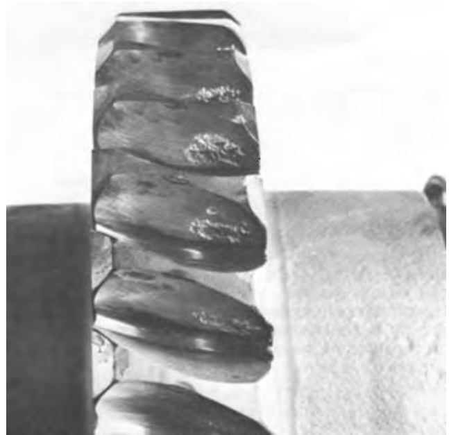
FIG. 2.19 (1169-16) WORM GEAR PITTING)
