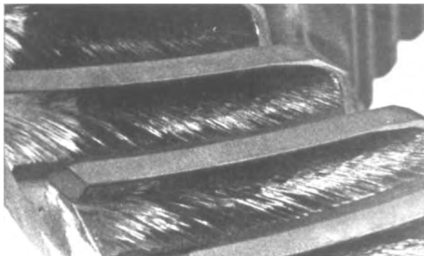
FIG. 2.39 (2342-18C) RIDGING
